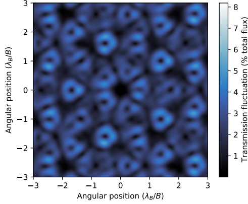
(b) Kernel 2
